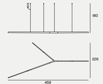
DIMENSIONS 459X226X8H - XL C MAXI
