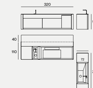
M1 320X150X93H / M2 220X72X93H
