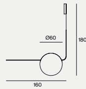
DIMENSIONS 160X180 - Ø40+Ø20
