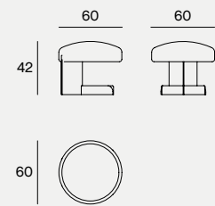
DIMENSIONS Ø 50X42H
