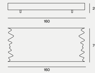
DIMENSIONS 160X70X20H
